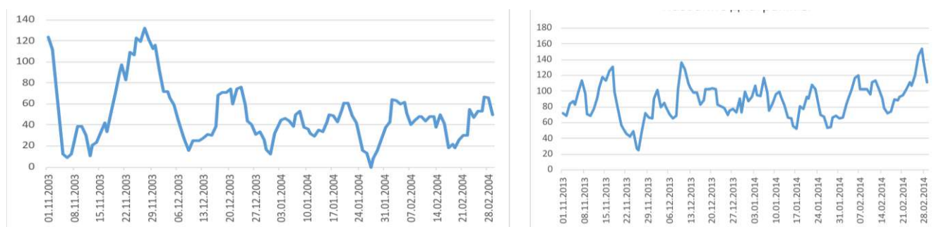
Рис. 9. Числа Вольфа в ноябре 2003-феврале 2004 и в ноябре 2013-феврале 2014
