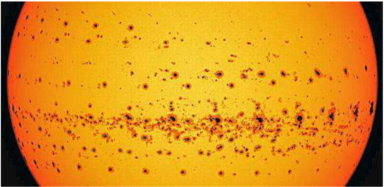
Рис. 12. Места на Солнце, где были пятна в обеих полушариях
