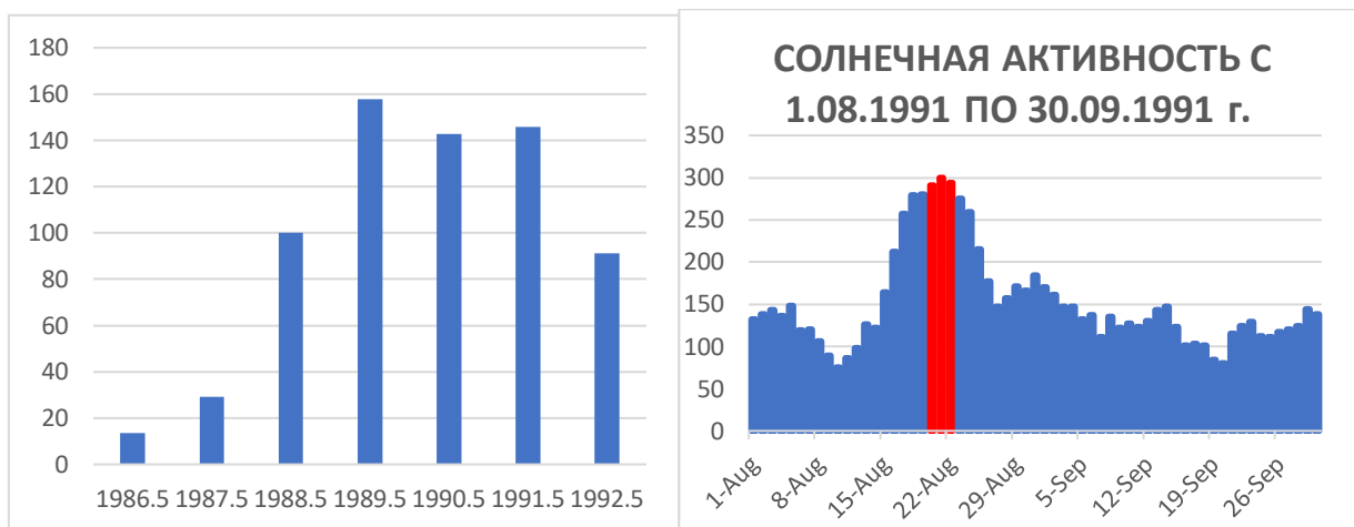
Рис. 1. Среднегод числа Вольфа с 1986 Рис. 2. Ежеднев числа Вольфа авг 1991
