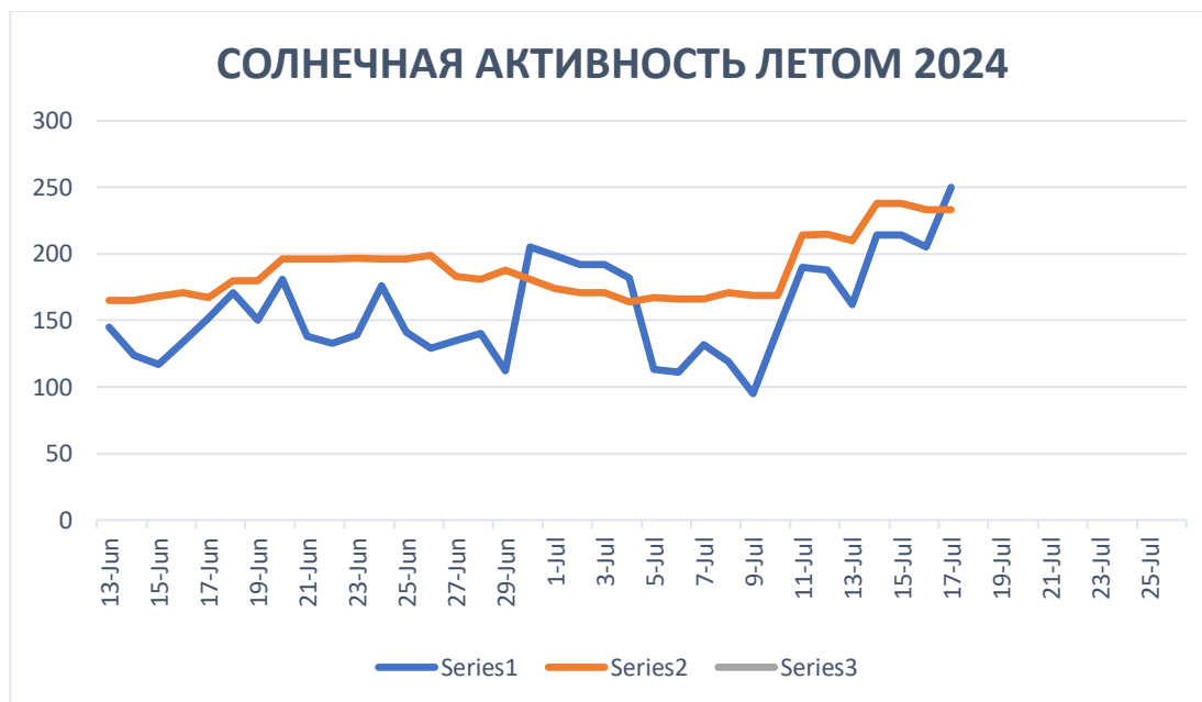
Рис. 10. Числа Вольфа (синяя) и интенсивность радиопотока Солнца на волне 10,7 см (красная)
