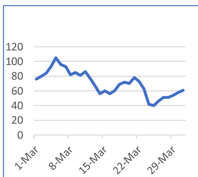
Рис. 4. Числа Вольфа в марте 1993 Рис.5.Числа Вольфа в сент – октябре 1993
